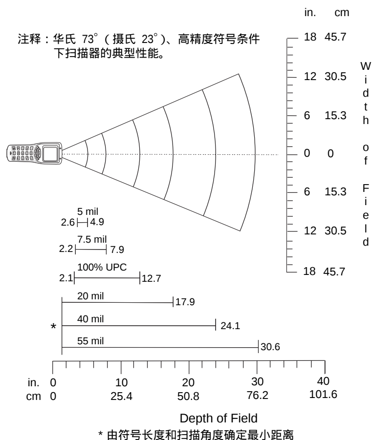
图 2-10 MC1000 激光解码范围
