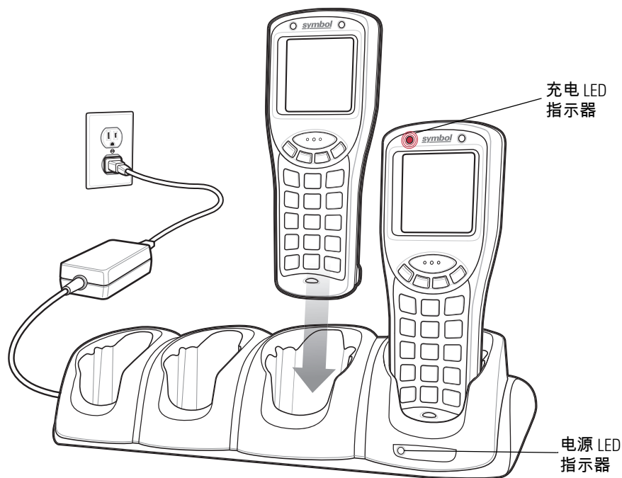
图 3-2 四槽 USB 通讯座
