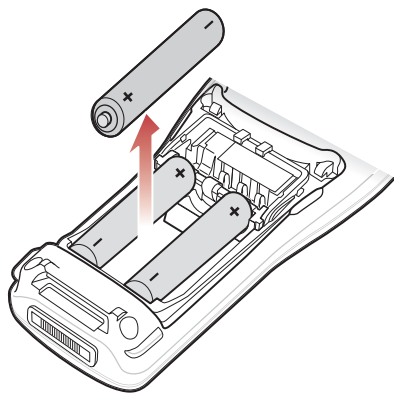
图 1-7 取出 AAA 电池
