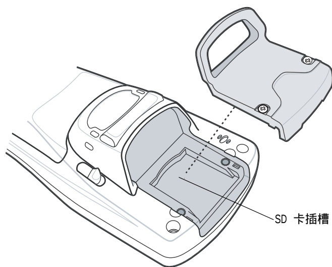
图 1-9 取出 SD 卡盖
