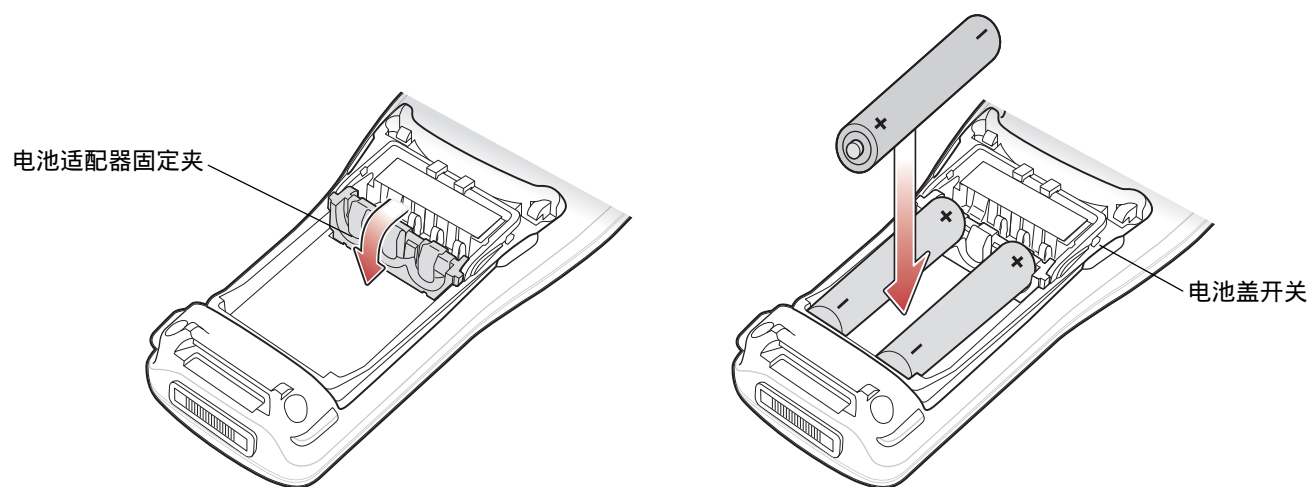
图 1-4 安装 AAA 电池
