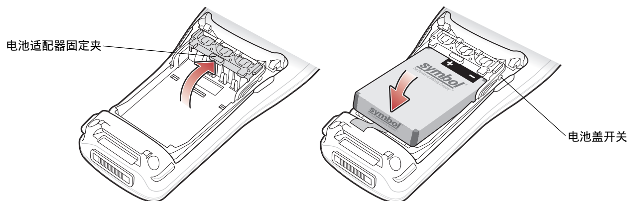
图 1-3 插入锂电池
