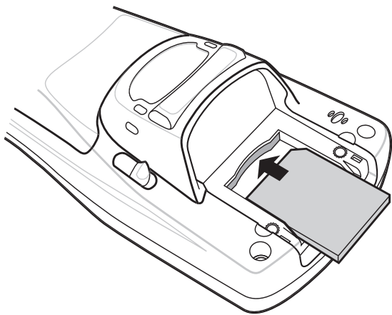
图 1-10 安装 SD 卡
