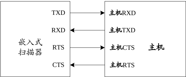
图 2-3 扫描器与主机的 RS-232 互连
