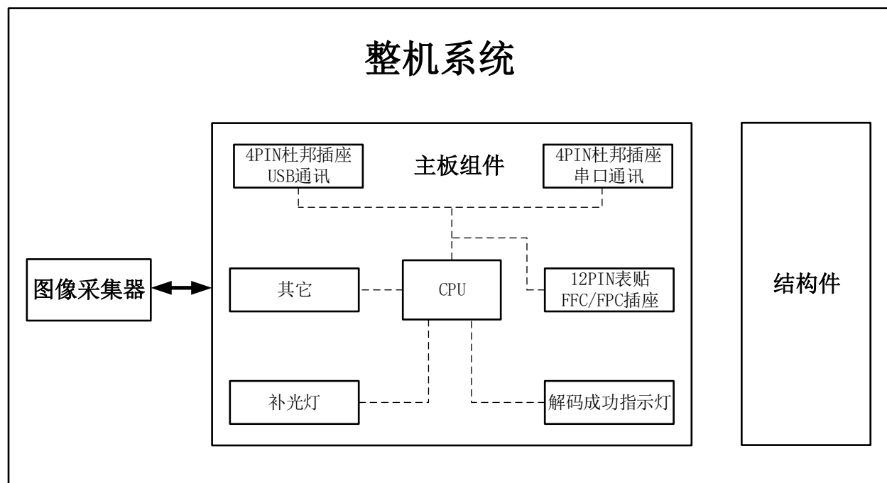
图 1-1 系统模块图：
