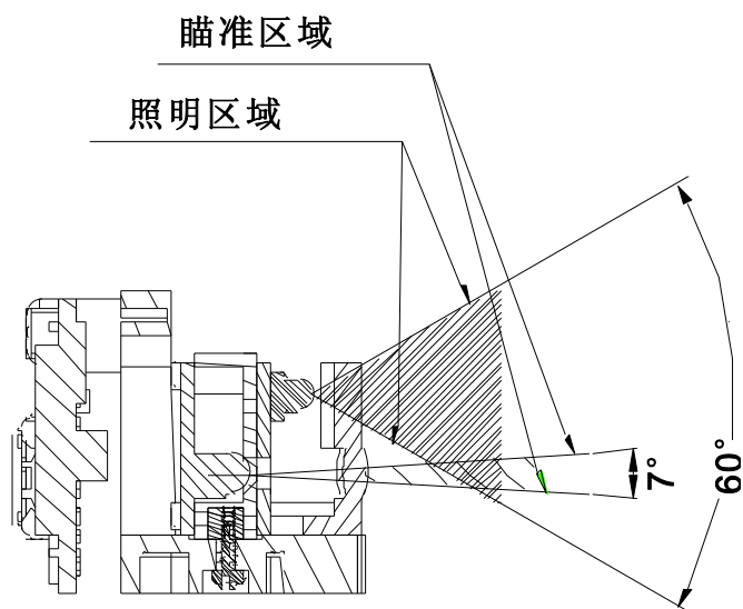
图 2-4 纵向切面
