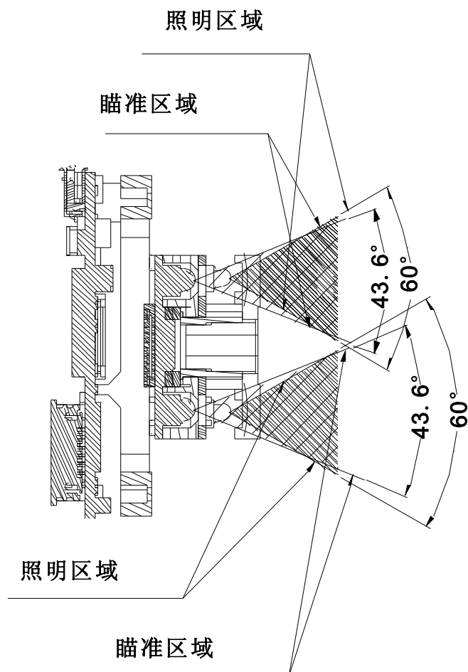
图 2-3 横向切面
