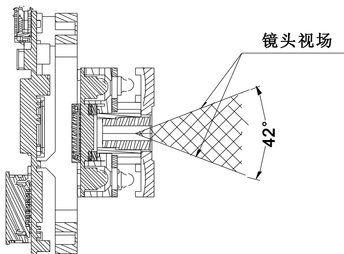
图 2-5 横向切面
