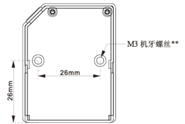
底视图
