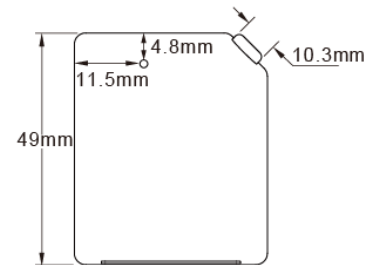
俯视图
