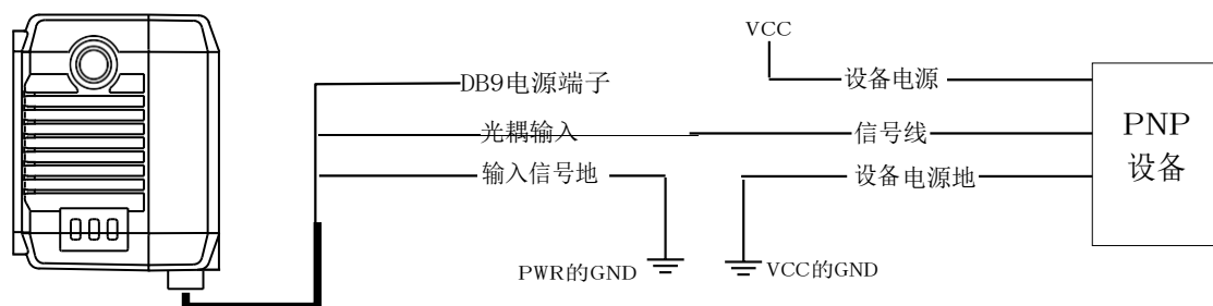
图4-5 输入信号接 PNP 设备
