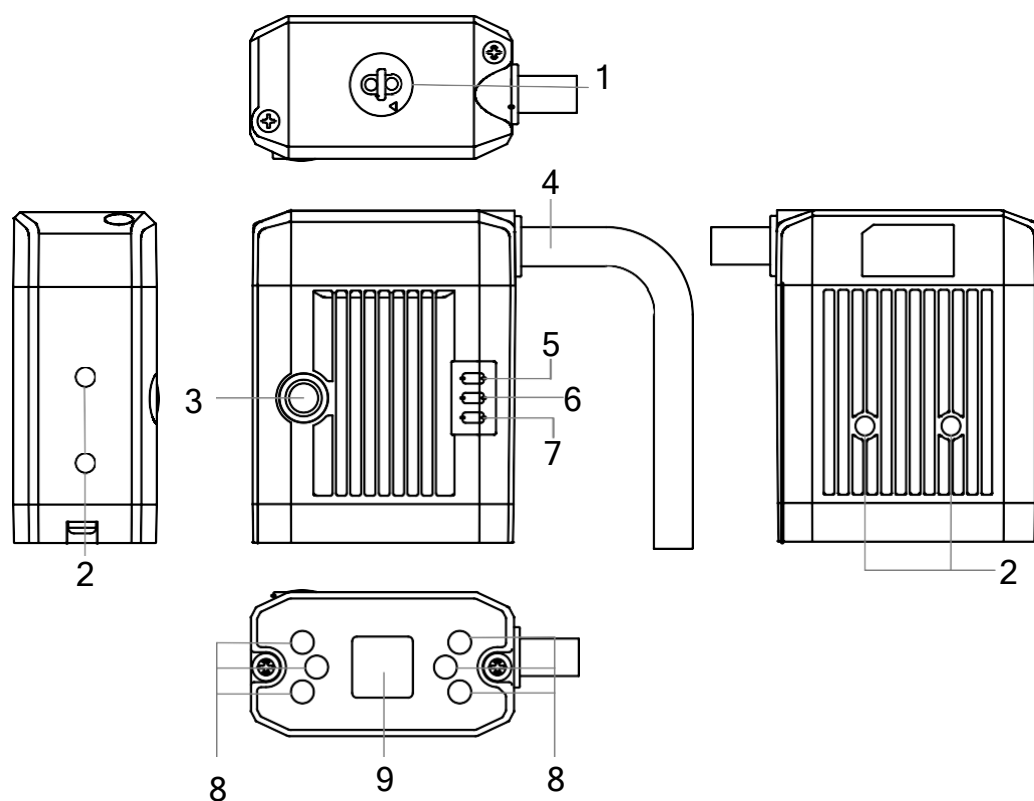
图1-3 手动调焦长焦，专用型设备外观
