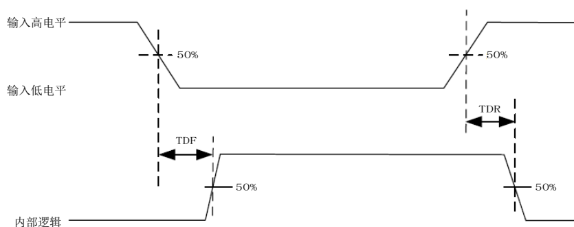
图4-2 输入逻辑电平
