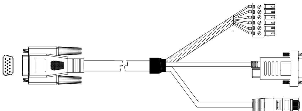
图1-12 DB15 线缆-RJ45 版
