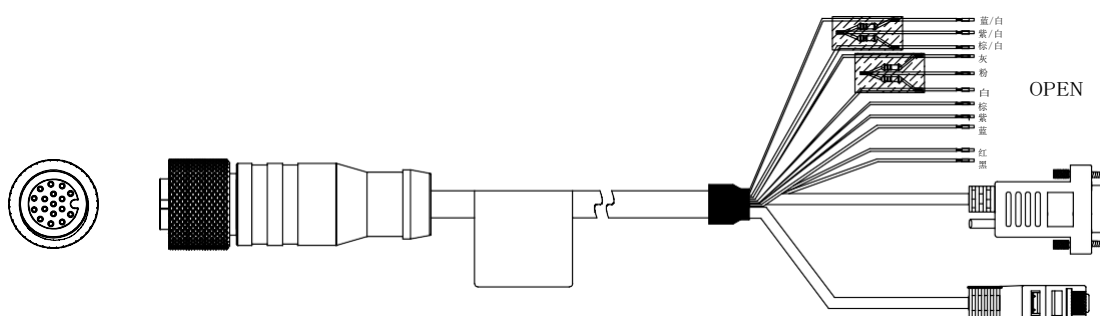
图1-8 17-pin M12 线缆-RJ45 版（手动调焦短焦、定焦设备使用）
