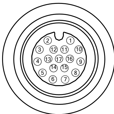
图1-9 17-pin 接口
