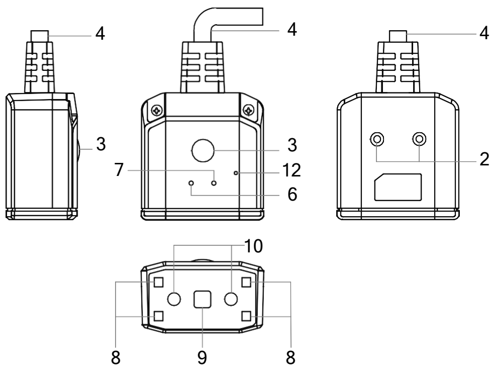
图1-6 定焦，经济型设备外观
