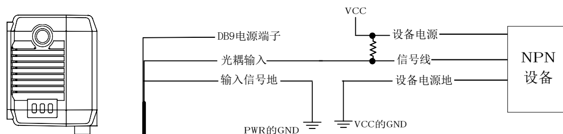
图4-7 输入信号接 NPN 设备（使用外接上拉电阻）
