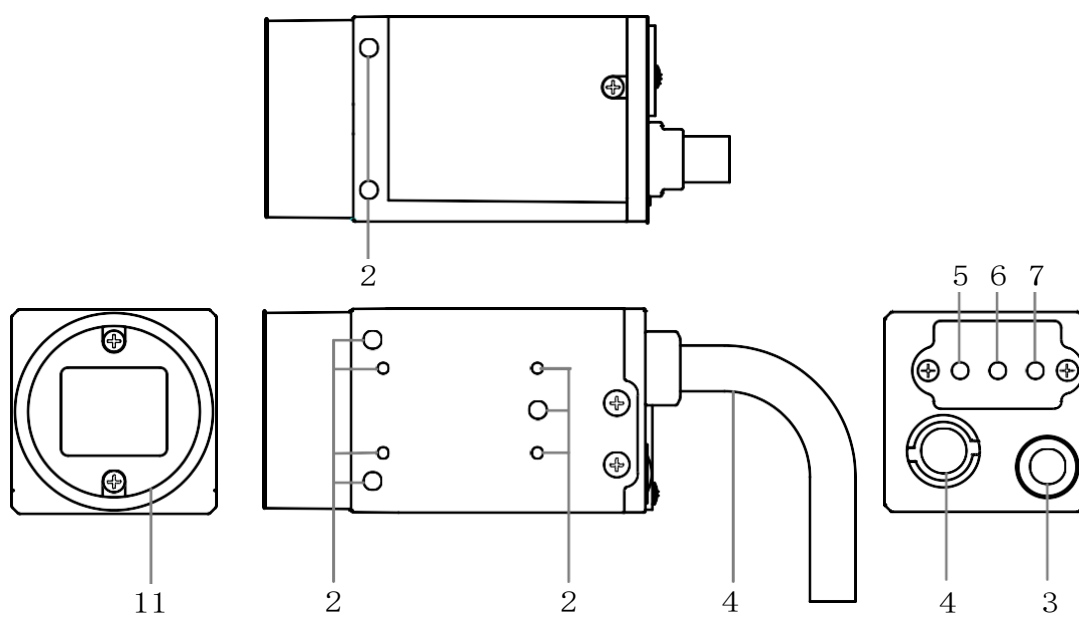
图1-4 C口专用型设备外观
