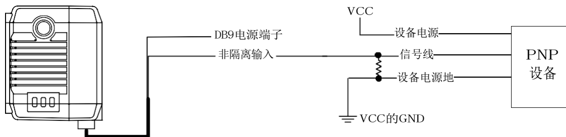
图4-19 输入信号接 PNP 设备（使用外接下拉电阻）
