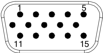
图1-11 DB15 接口
