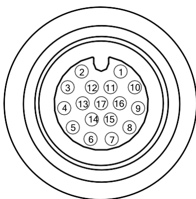
图1-7 17-pin 接口
