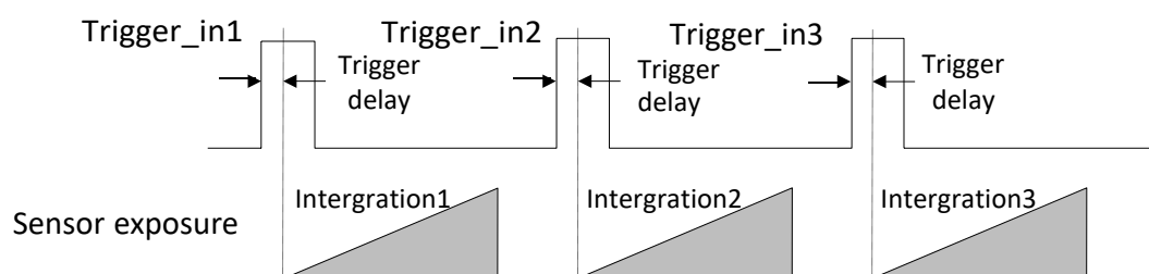
图3-34 信号延迟原理
