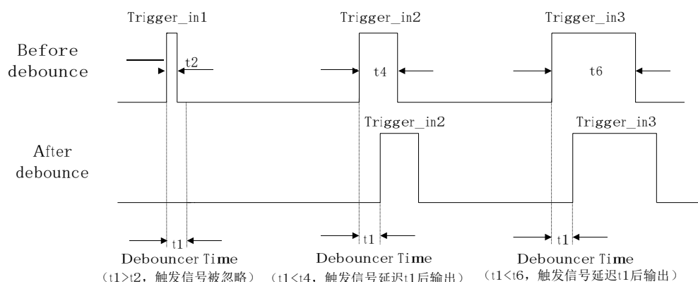
图3-36 触发输入信号去抖时序
