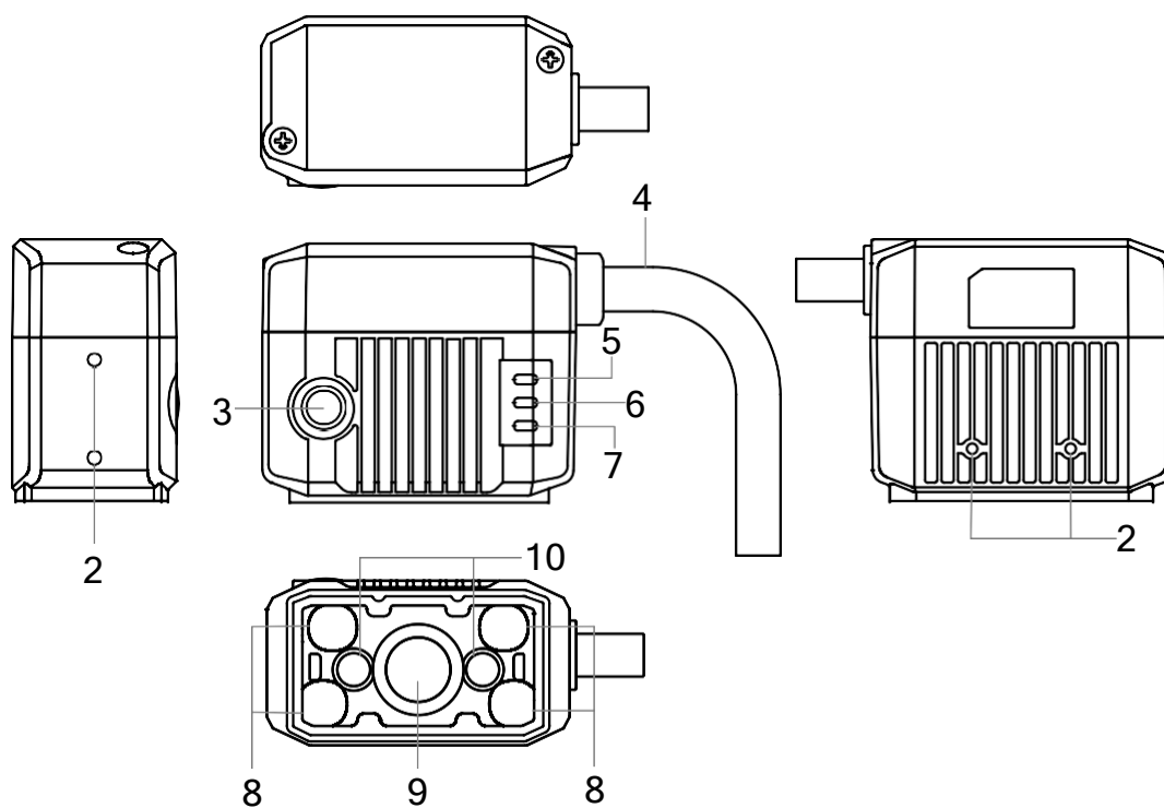
图1-1 固态调焦，专用型设备外观
