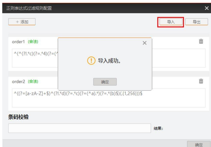
图3-59 正则表达式过滤规则导入
