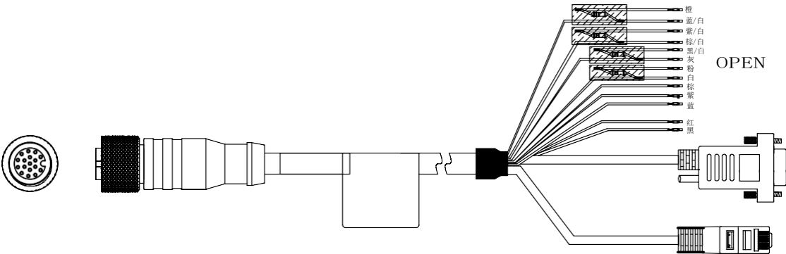
图1-10 17-pin M12 线缆-RJ45 版（其他专用设备使用）
