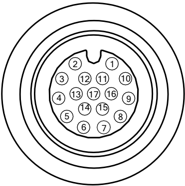
图1-14 17-pin 接口
