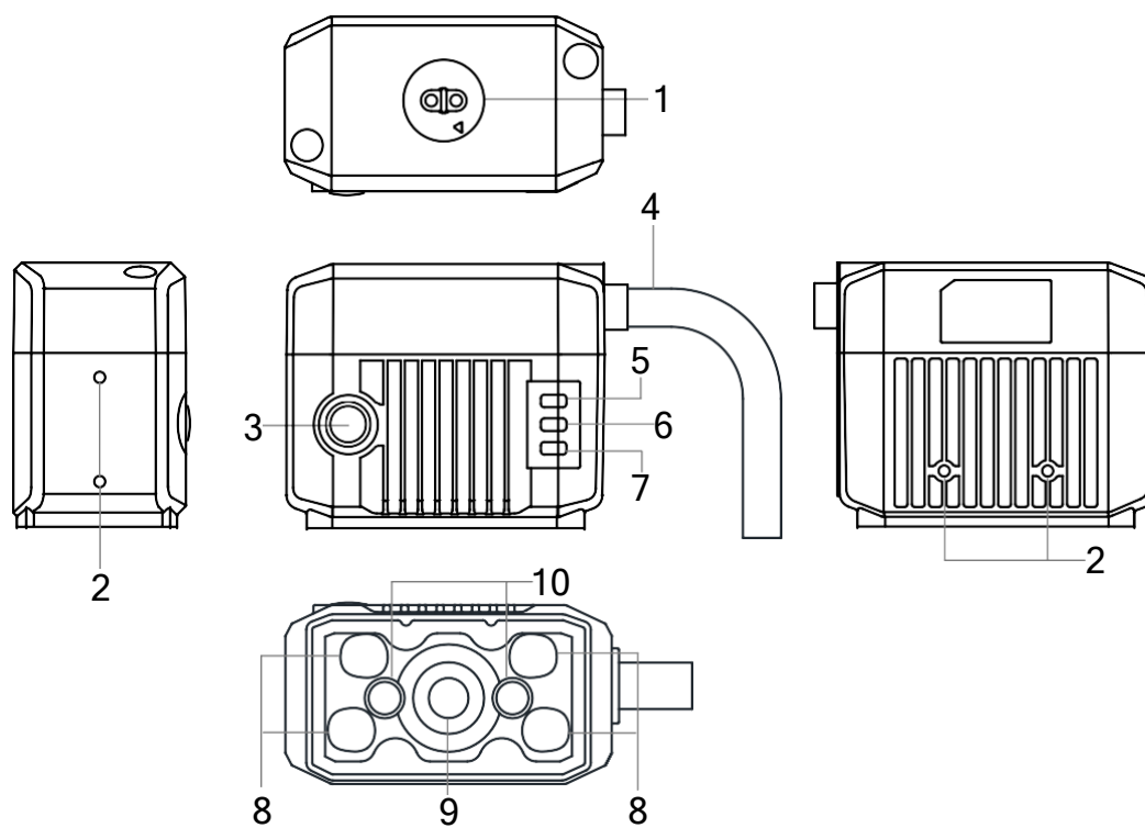
图1-2 手动调焦短焦，专用型设备外观
