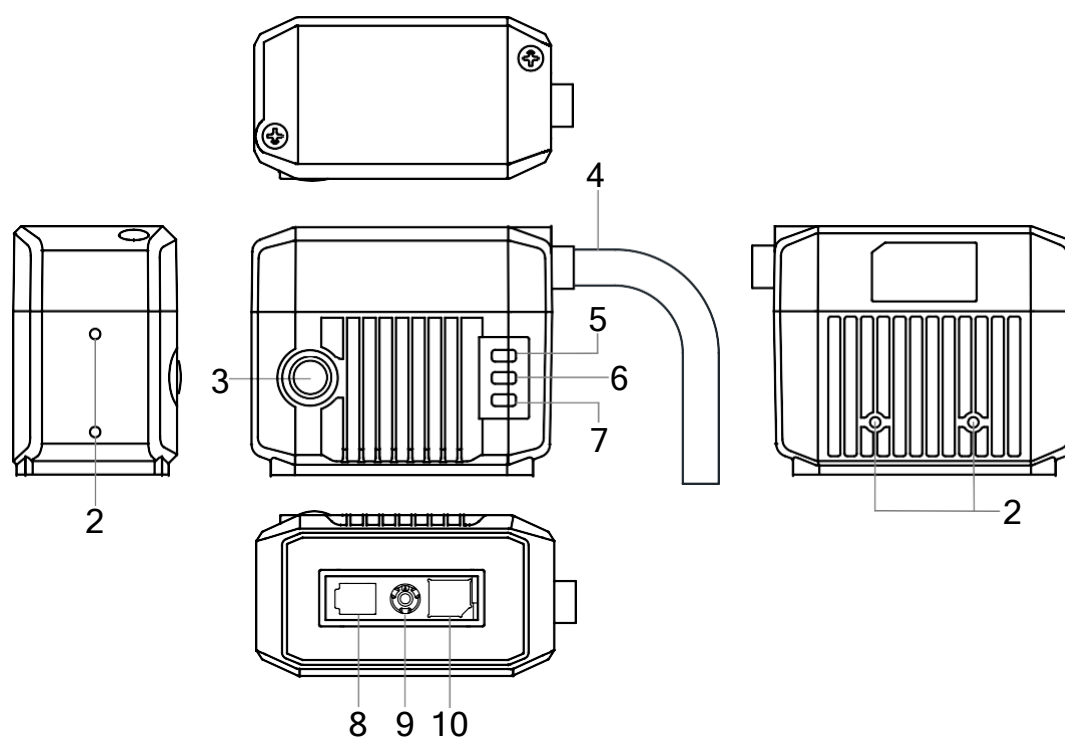
图1-5 定焦，专用型设备外观
