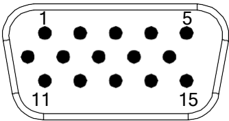
图1-16 DB15 接口
