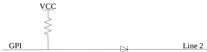
图4-11 Line 2 内部电路
