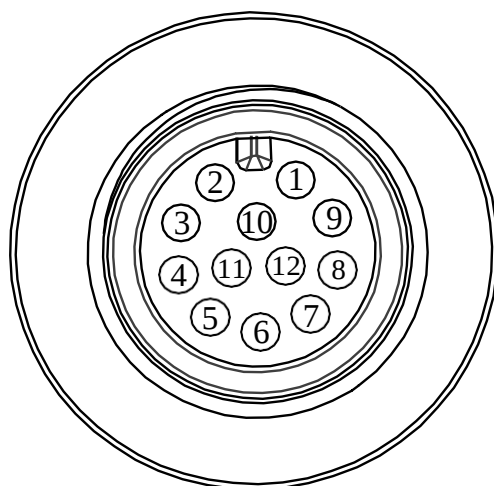
图1-5 12-pin M12 接口
