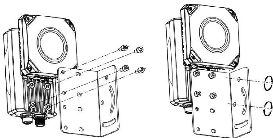
图2-2 正面安装
