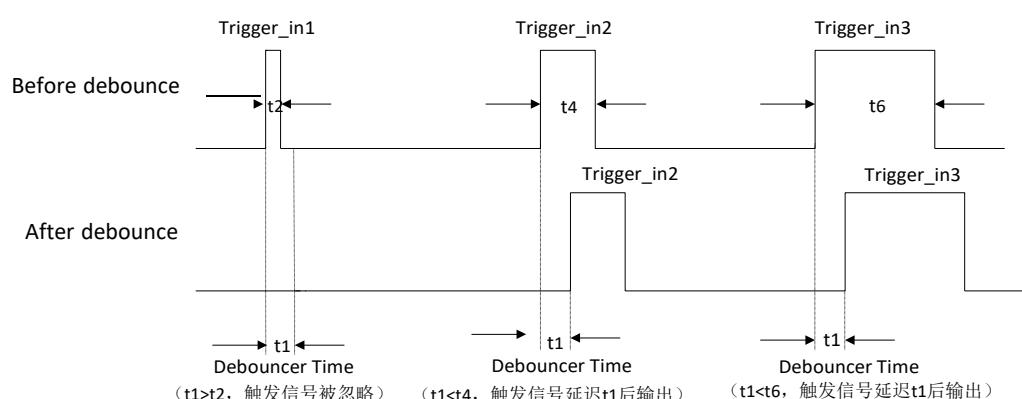
图3-46 触发输入信号去抖时序
