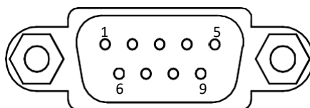
图4-11 9-pin 公头连接器
