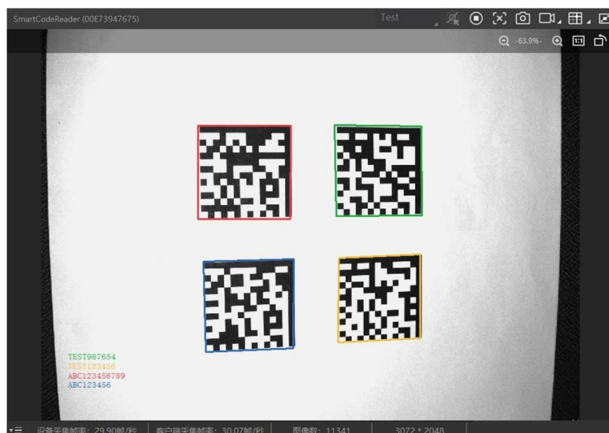
图2-12 设备实时预览
